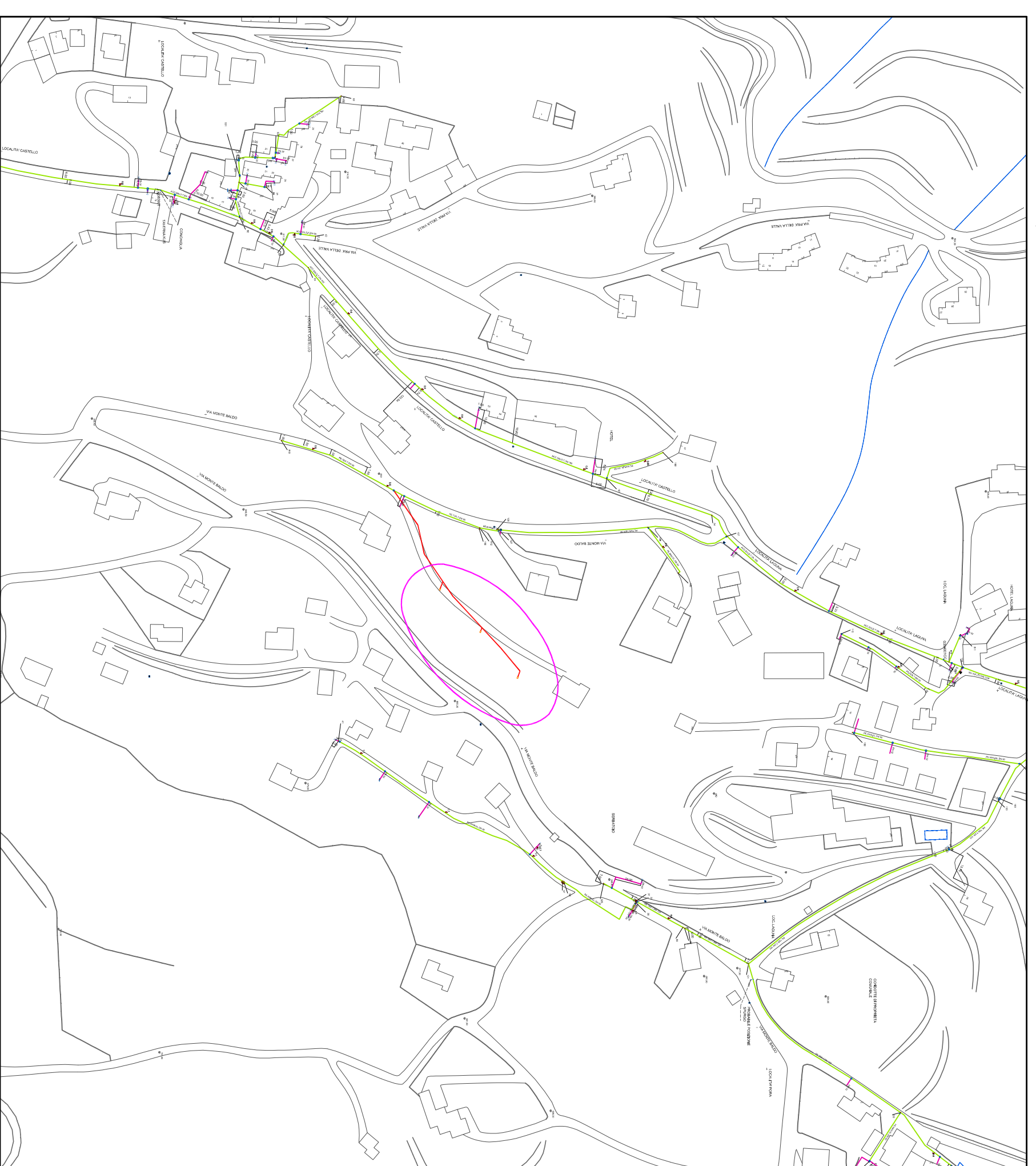
CARTOGRAFIA TECNICA REGIONALE VENETO scala 1:2500 Comune di SAN ZENO DI MONTAGNA Provincia di VERONA CON INDICAZIONI RETE GAS ESISTENTE E IN PROGETTO
