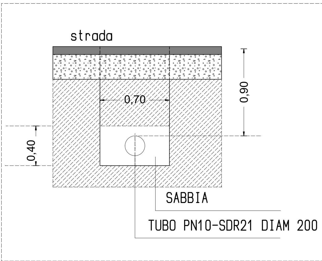
CONDOTTA FOGNARIA
