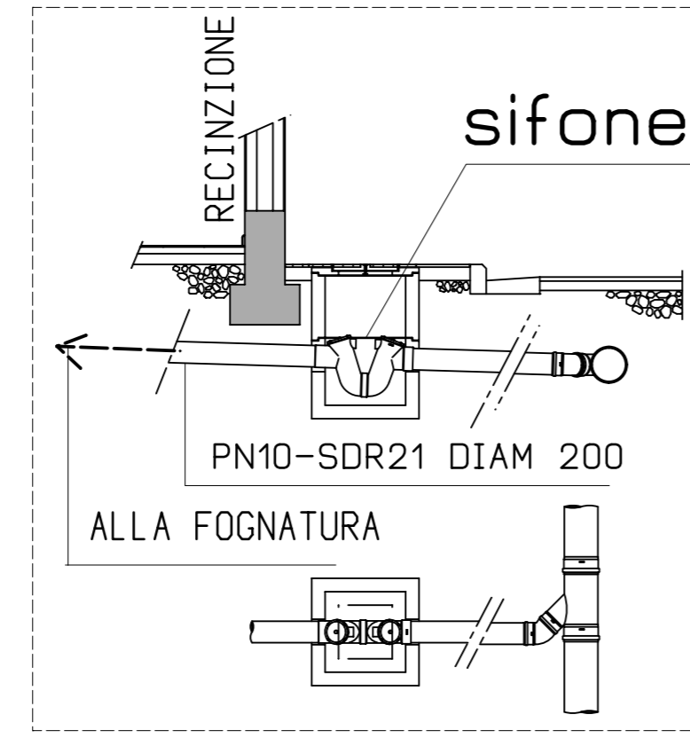
SIFONE
